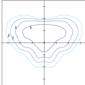
ISO Footcandle
