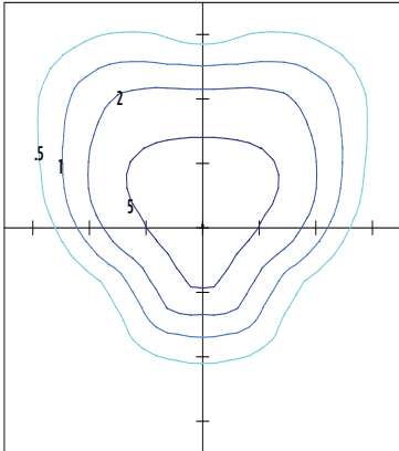
ISO Footcandle
