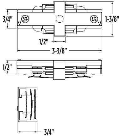
Mini Connector
