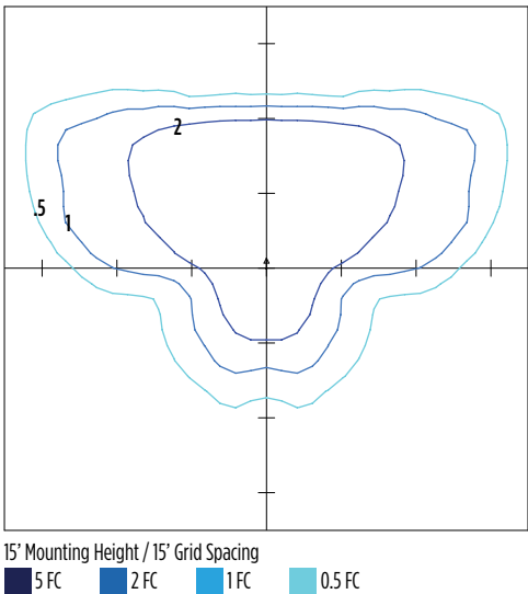
ISO Footcandle
